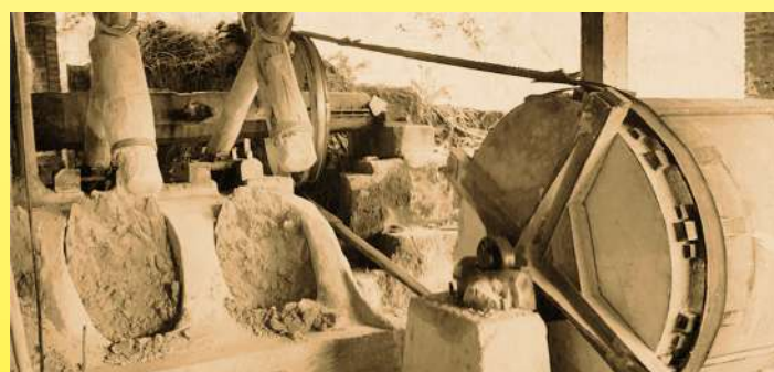
Herkömmliche Produktionsmaschinen (( 水碓 shuǐ duì) zur Erzeugung von Pulvern für die Herstellung von Elektroporzellan (Privatsammlung)
